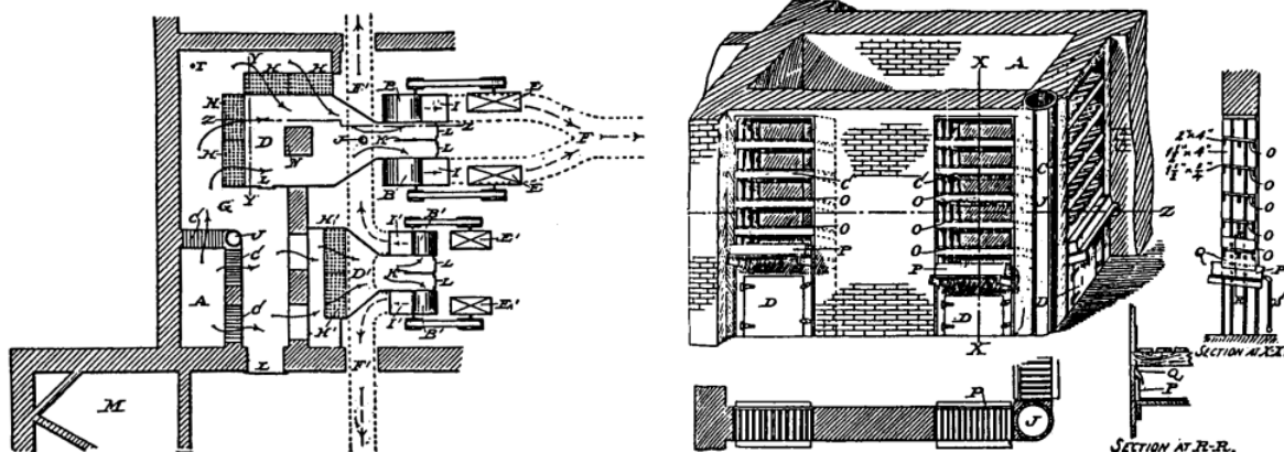
図 カーネギーホールの機械室（参考文献3））図 カーネギーホールの氷柵（参考文献3））
