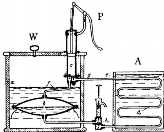
図 パーキンスのエーテル機（参考文献3））
