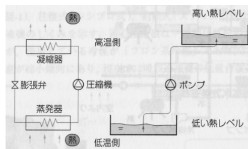
図 冷凍サイクルとヒートポンプ（参考文献1）
