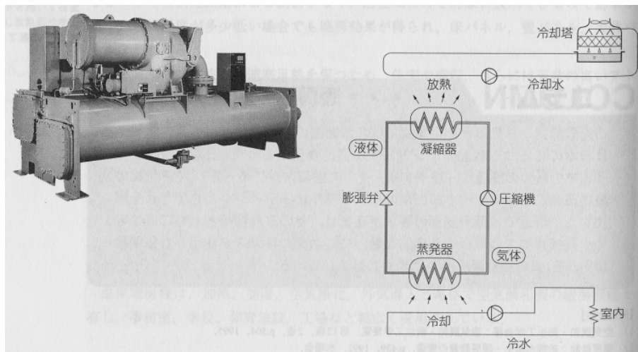
図 遠心（ターボ）冷凍機（参考文献1） 図 圧縮式冷凍機のしくみ（参考文献1）
