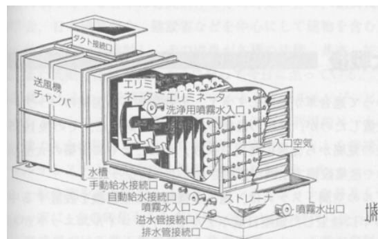
図 エアワッシャー（参考文献1）
